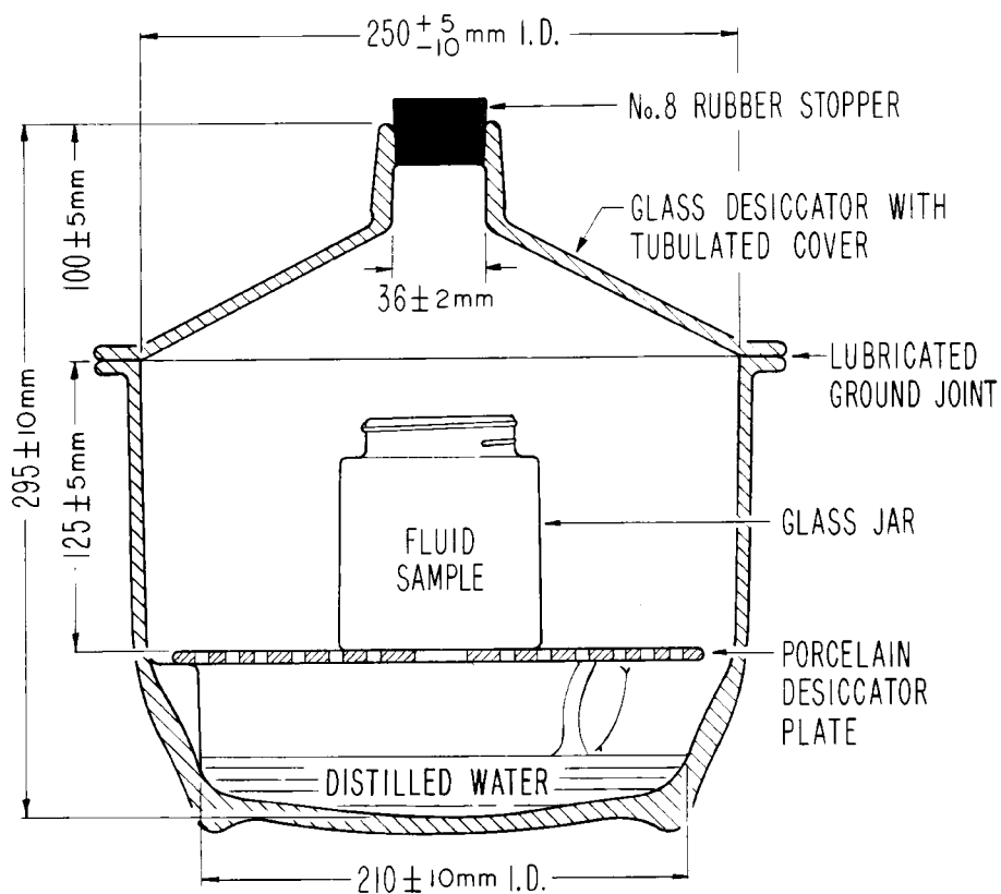
FIG. 3 HUMIDIFICATION APPARATUS
